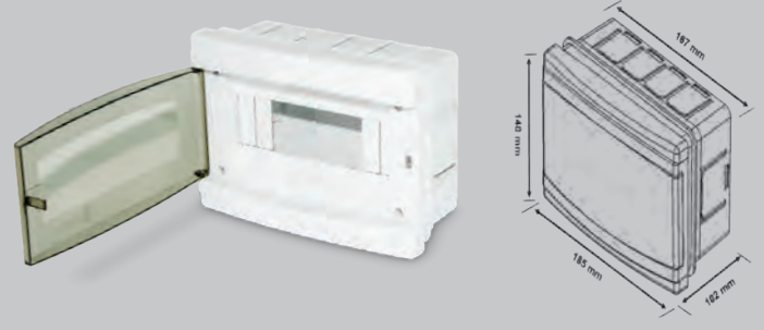
6'lı Siva Altı Sigorta Kutusu 6 Module Distribution Box - Recessed
